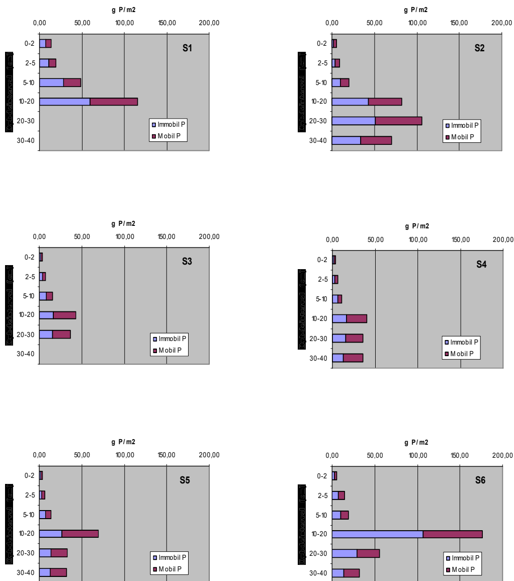
Figur 3. Puljer af immobilt og mobilt P i de enkelte dybdeintervaller på de 6 stationer i Søllerød Sø. Bemærk at enheden er "g P m -2 ". Lagtykkelsen af de pågældende dybdeintervaller er derfor medregnet i værdierne.
