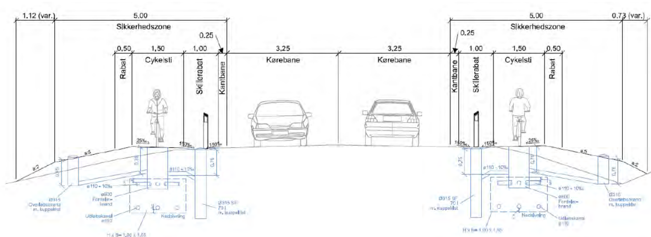
Principsnit af rockflowanlæg langs Hørsholm Kongevej
