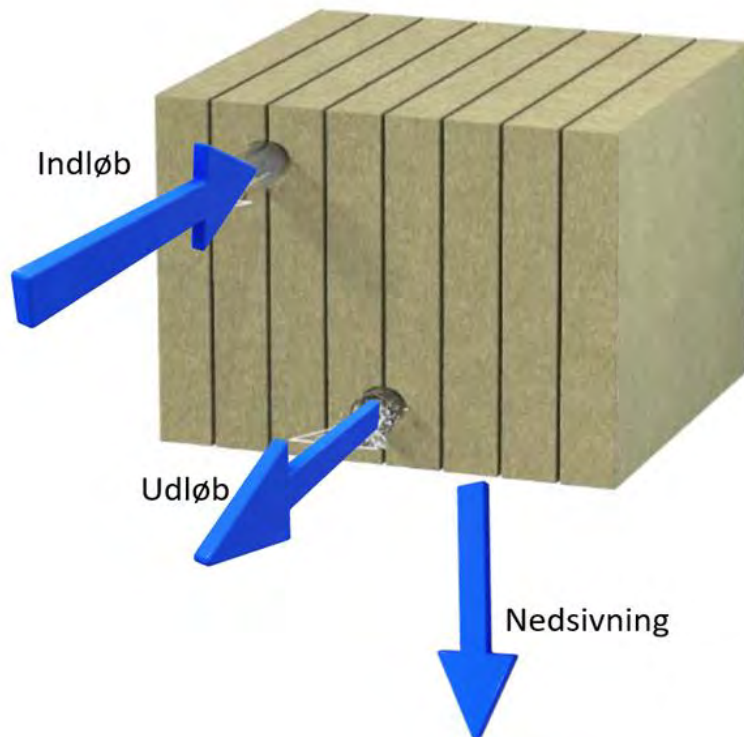
Figur 5-5. Principskitse af Rockflow-modul. Regnvandet løber ind via fordelingskanalen foroven, siver ned gennem anlægget og enten udlødes eller nedsives. Efter (WSP, 2023).
