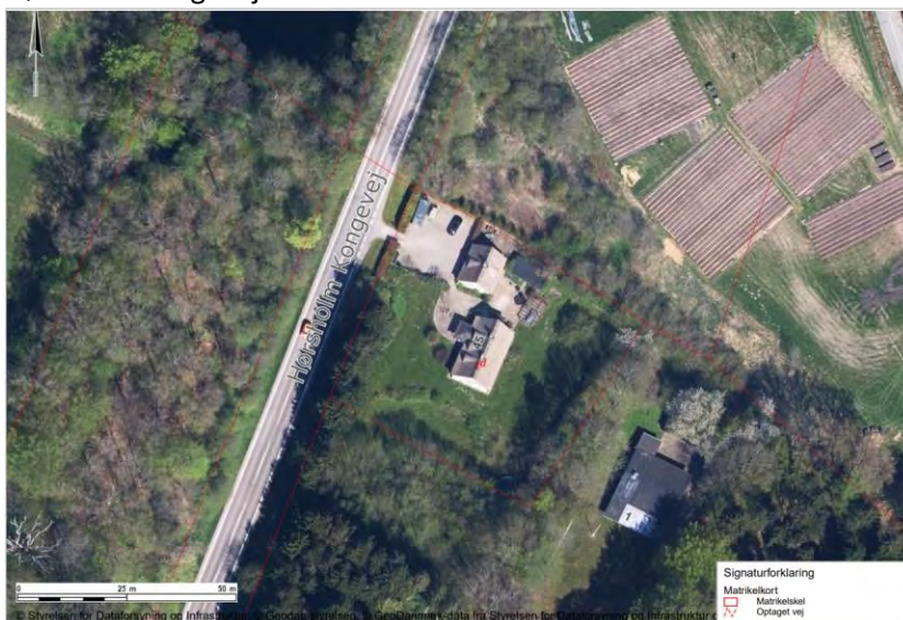
Figur 18 Matrikelkort ( https://sdfikort.dk/spatialmap )
