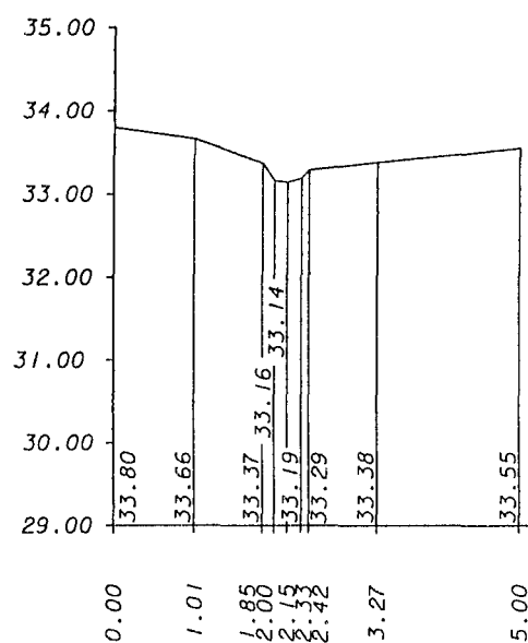
TVÆRPROFIL Station 727
