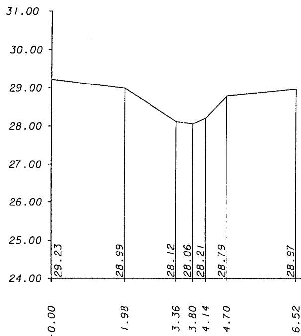
TVÆRPROFIL Station 2199
