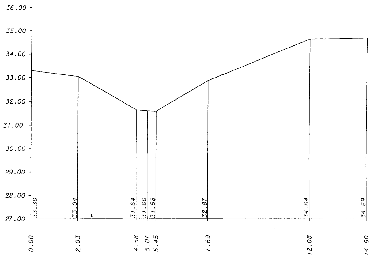
TVÆRPROFIL Station 1424
