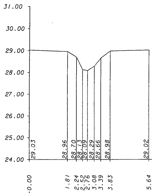
TVÆRPROFIL Station 1896
