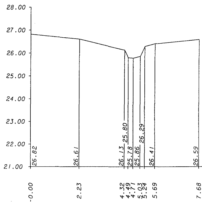
TVÆRPROFIL Station 2561
