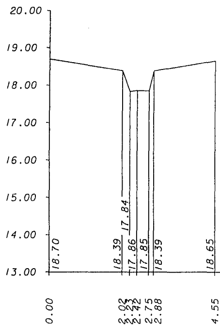
TVÆRPROFIL Station 3608
